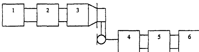
1 - шумомер; 2 - усилительно-питающее устройство; 3 - искусственное ухо; 4 - испытуемый ЦТА; 5 – блок сопряжения; 6 - генератор цифровых сигналов.
