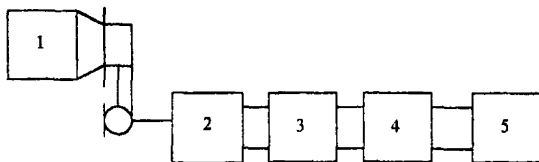
1 - искусственное ухо; 2 - испытуемый ЦТА, 3 – блок сопряжения; 4 - эталонный кодек; 5 – псофометр.
