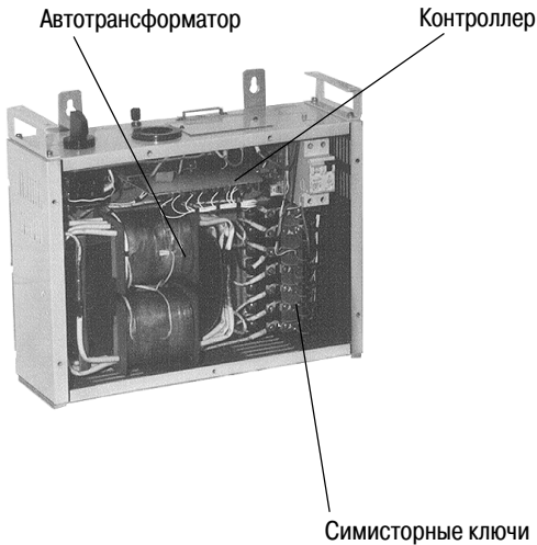
Рис. 8. Устройство стабилизатора
