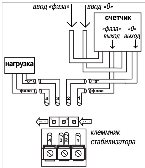
Рис. 17. Схема установки
